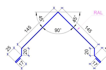
Планка карнизная ТИП 2
