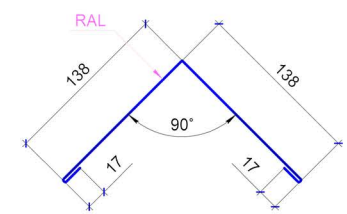
Планка карнизная ТИП 3
