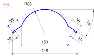
Планка ветровая ТИП 1
