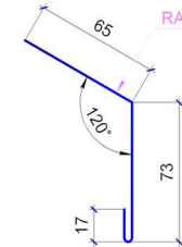
Планка ветровая ТИП 3
