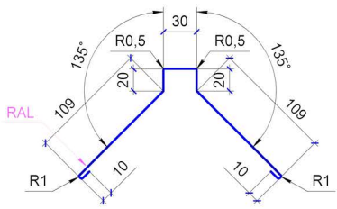
Планка конька ТИП 7
